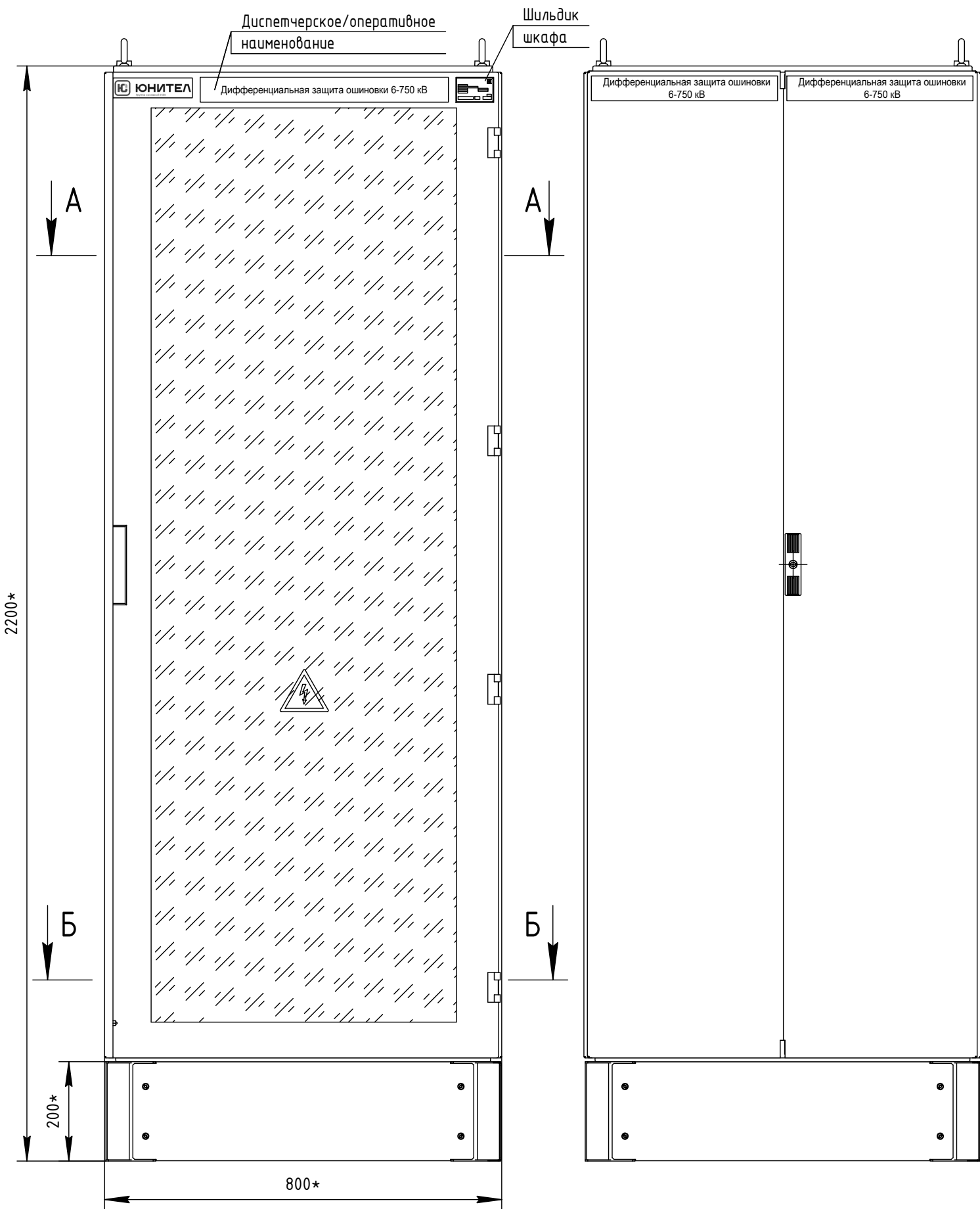
Вид сзади
