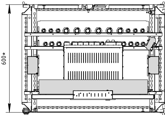
Б-Б
