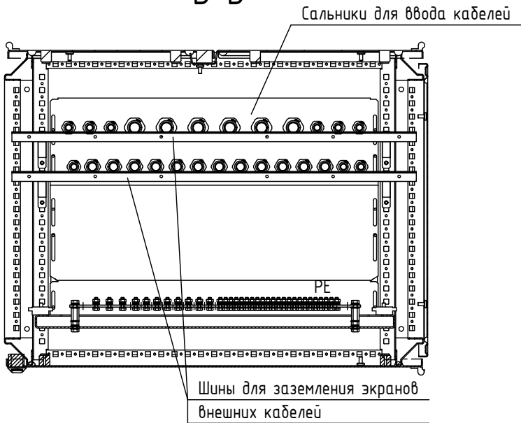
Б-Б
